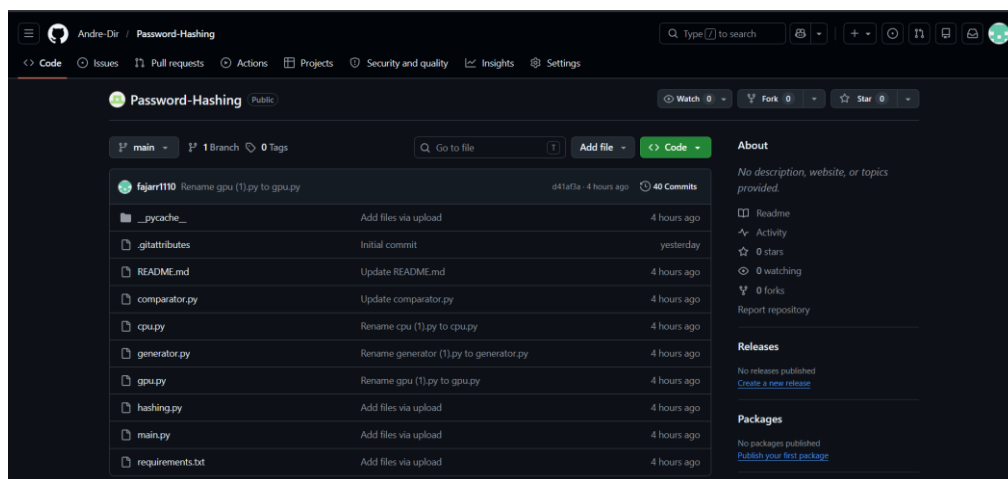
Gambar 7 Struktur Repository
